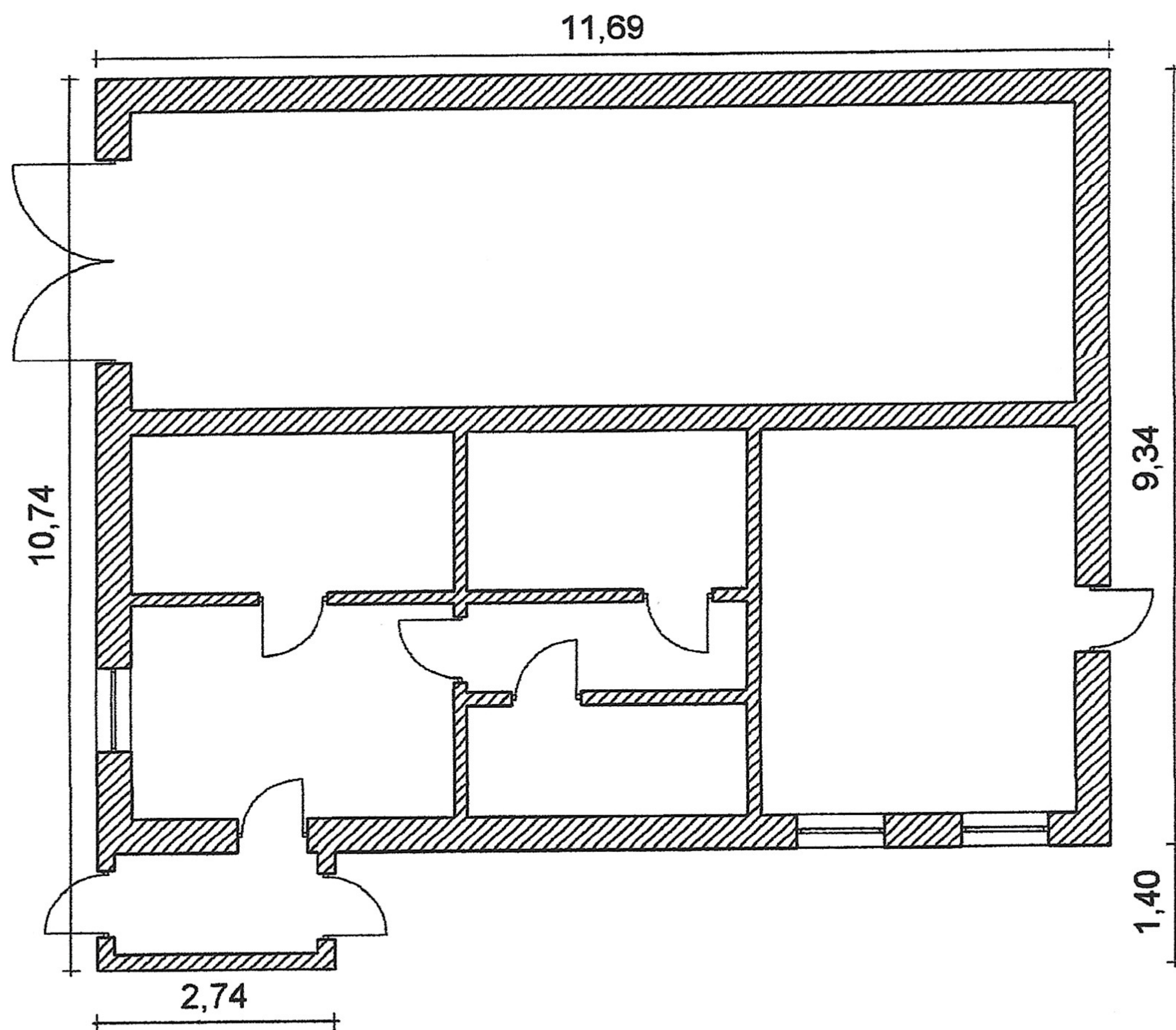
Pôdorys M 1:100
